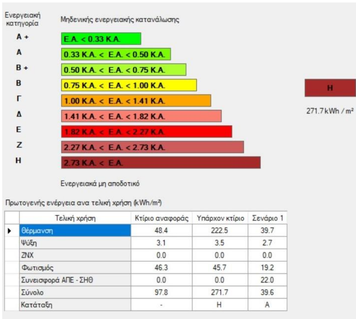
Εικόνα 17: Ενεργειακή Κατάταξη
